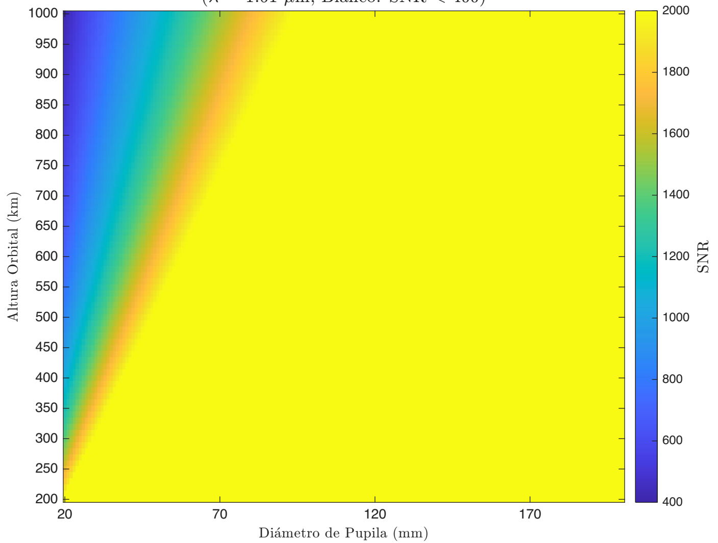
SNR - Refractivo - Detector 1 ( \lambda = 1.61 \mu\text{m} , Blanco: SNR < 400)
